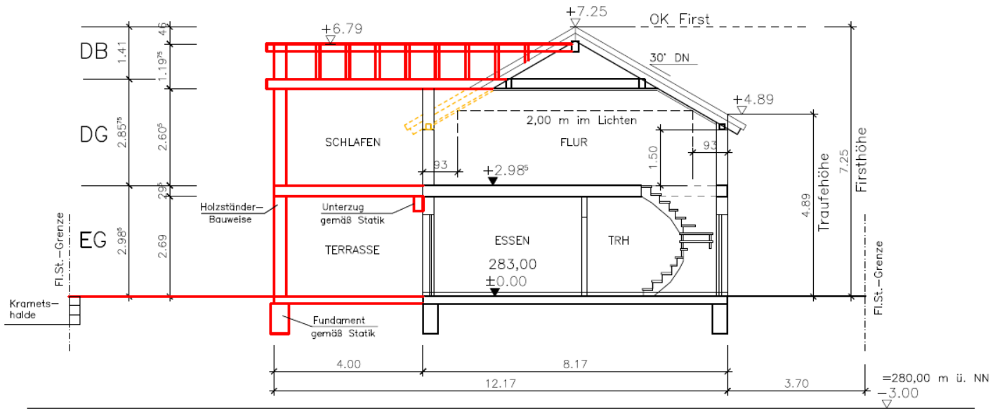
Schnitt A-A
