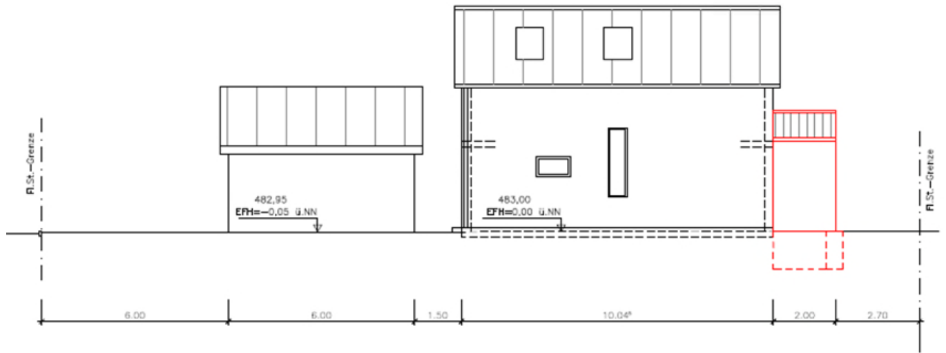
Ansicht Osten
