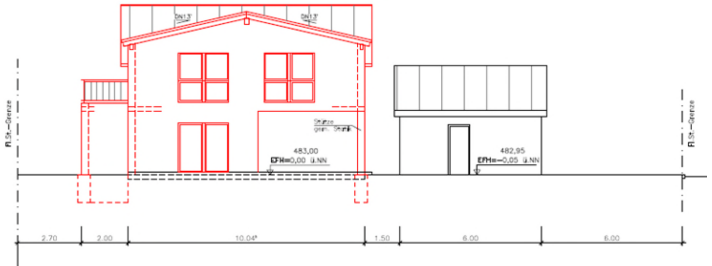
Ansicht Westen
